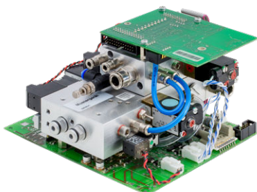
Digitaler Gasmischer
