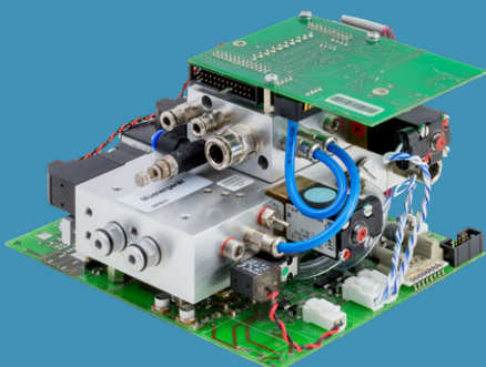
Digitaler Gasmischer
